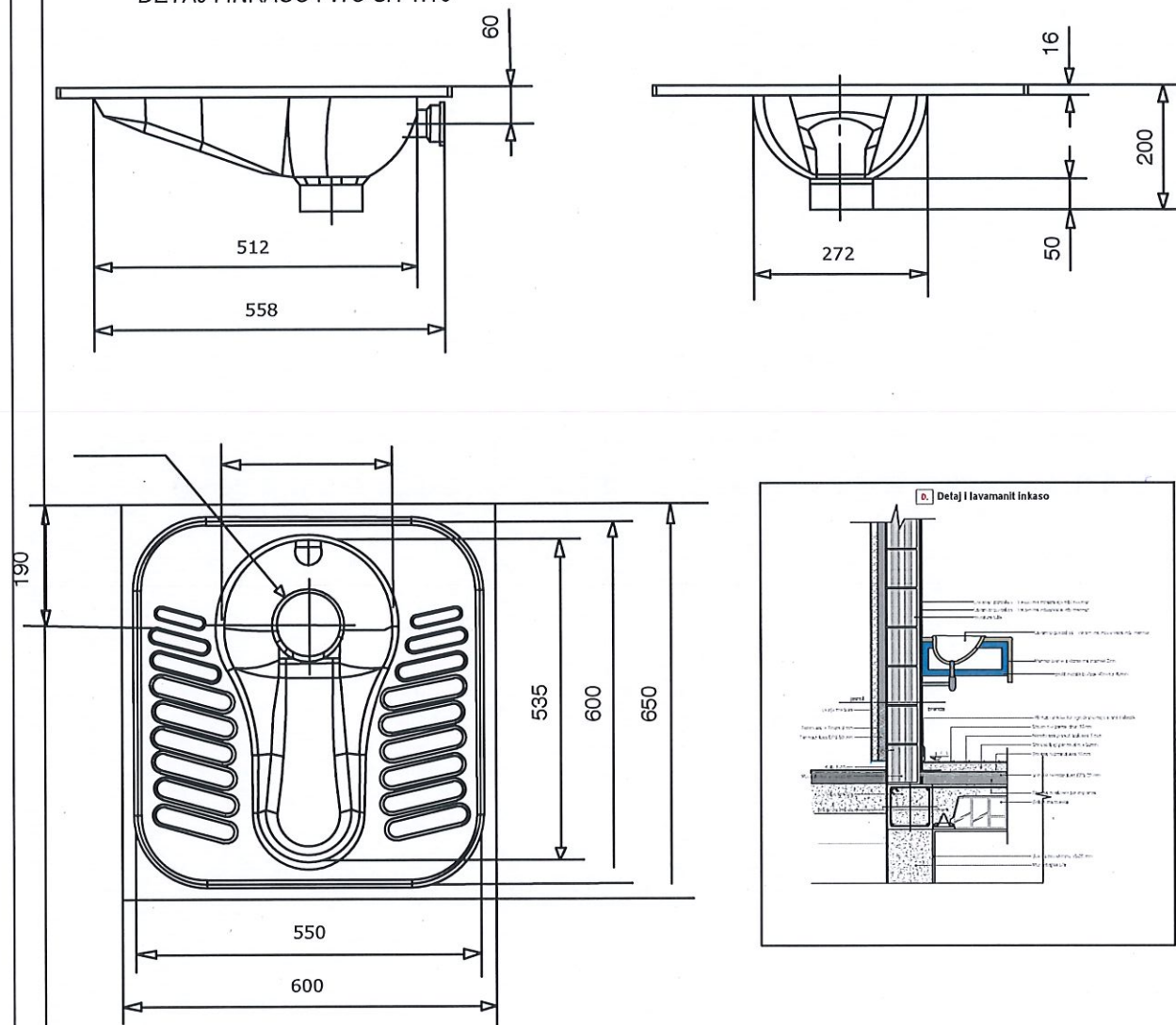
DETAJ I INKASO I WC SH 1:10
