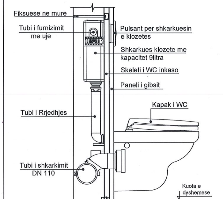
DETAJ I WC INCASO
