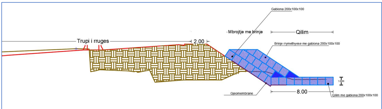
Profili Tip ne km 2+100 deri km 2+367
