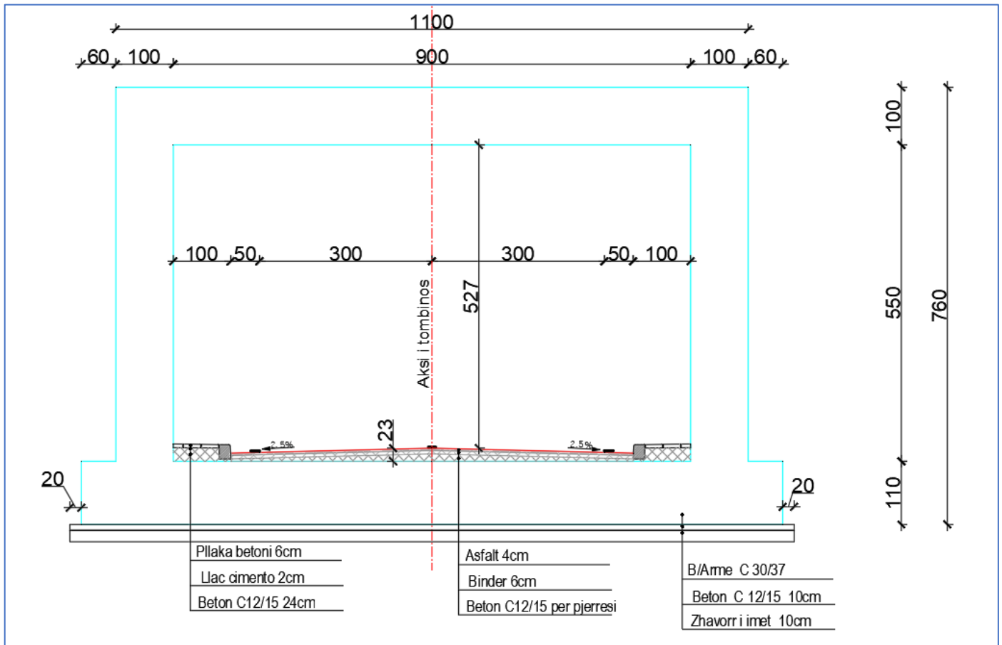
Profil Tip, Nenkalimi ne km 2+960 (Xibrake) dhe km 5+570 (Mirake)
