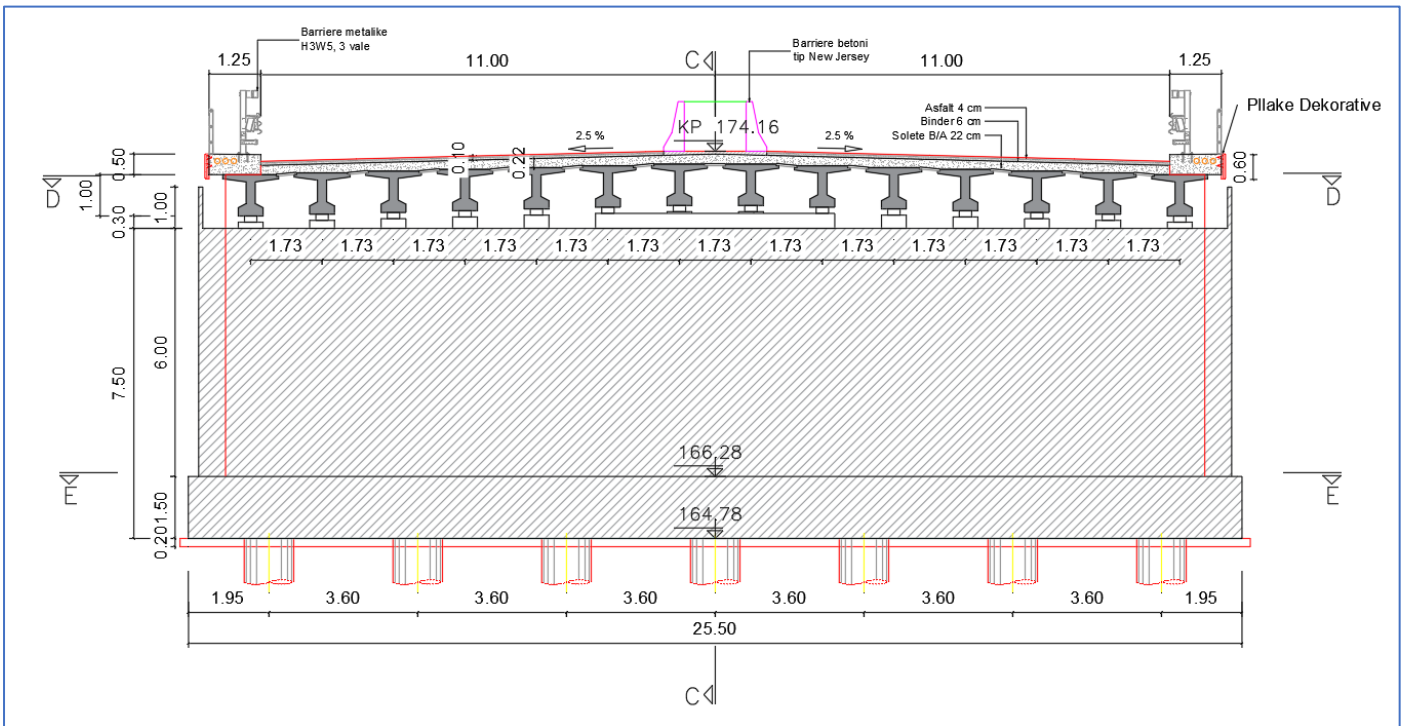
Profil Tip, Ura km 4+300
