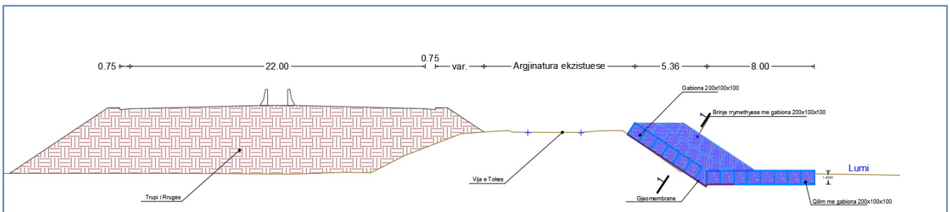
Profili Tip ne km 3+275 deri km 3+630
