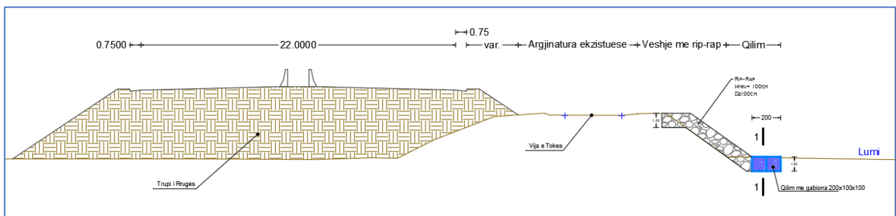
Profili Tip ne km 3+630 deri km 4+044
