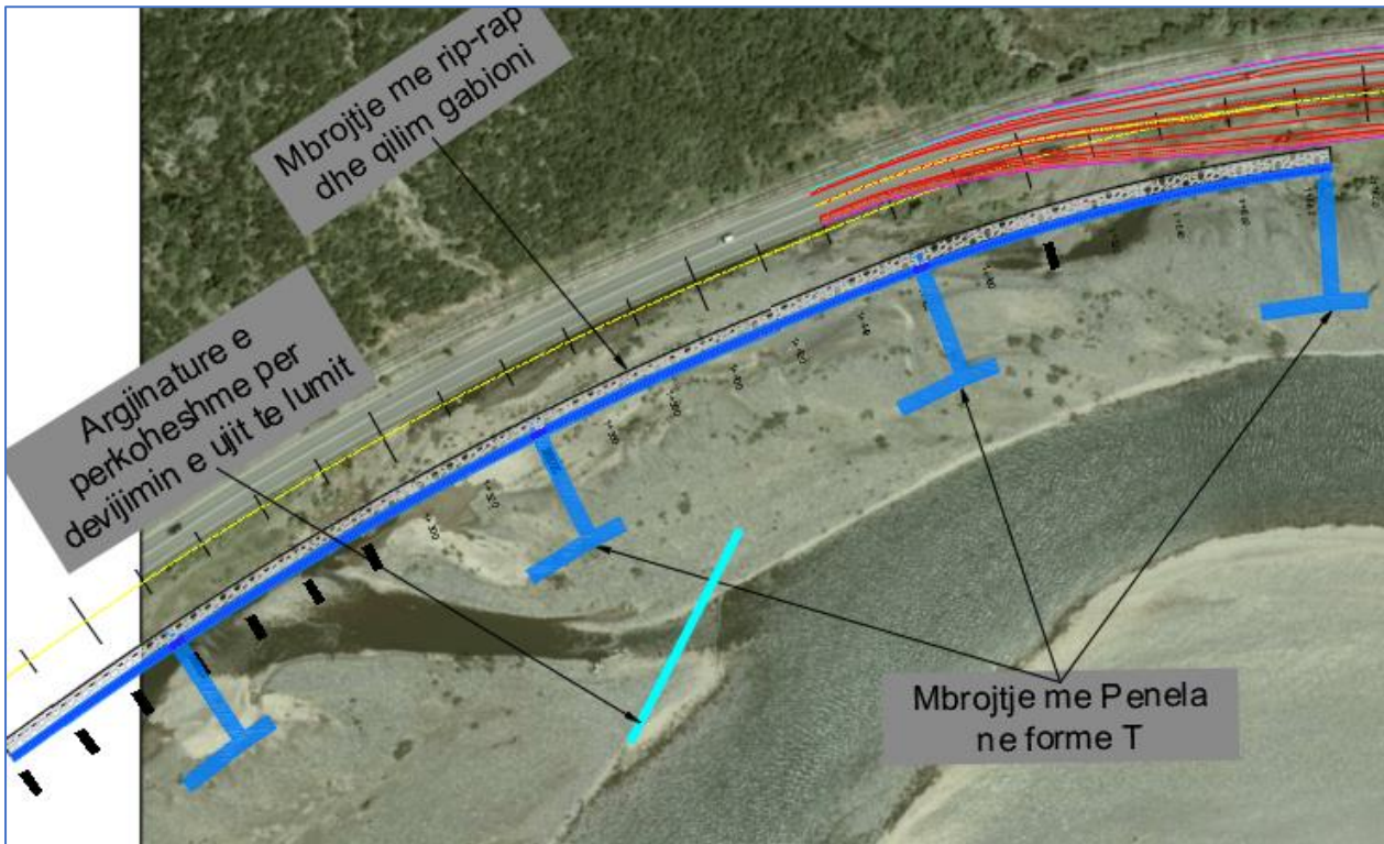
Mbrojtja Lumore ne km 1+440 ( fillimi i rruges )
