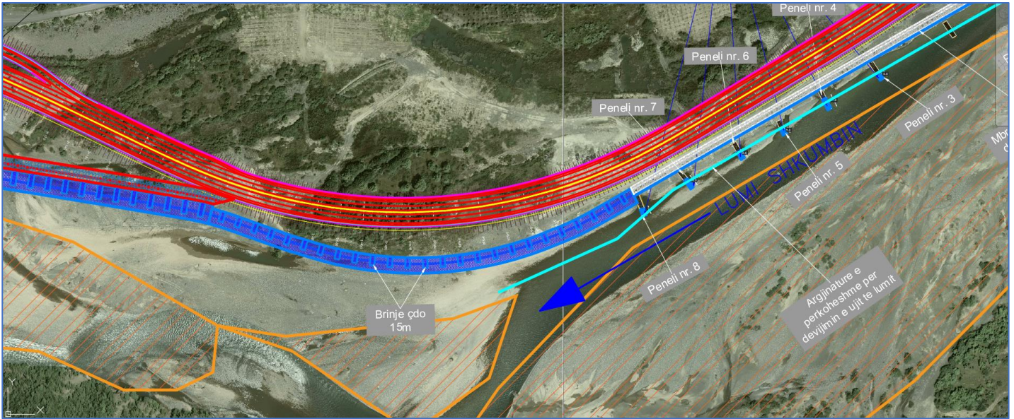
Planimetria e Mbrojtjes Lumore ne km 3+275 deri km 3+630
