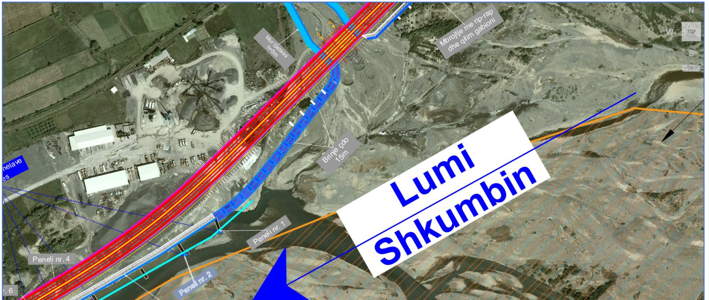
Planimetria e Mbrojtjes Lumore ne km 4+044 deri km 4+290
