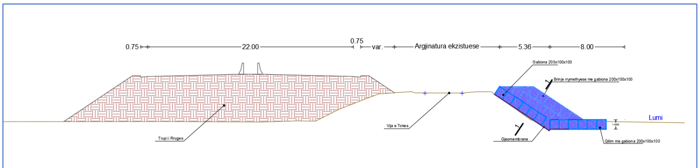
Profili Tip ne km 4+044 deri km 4+290
