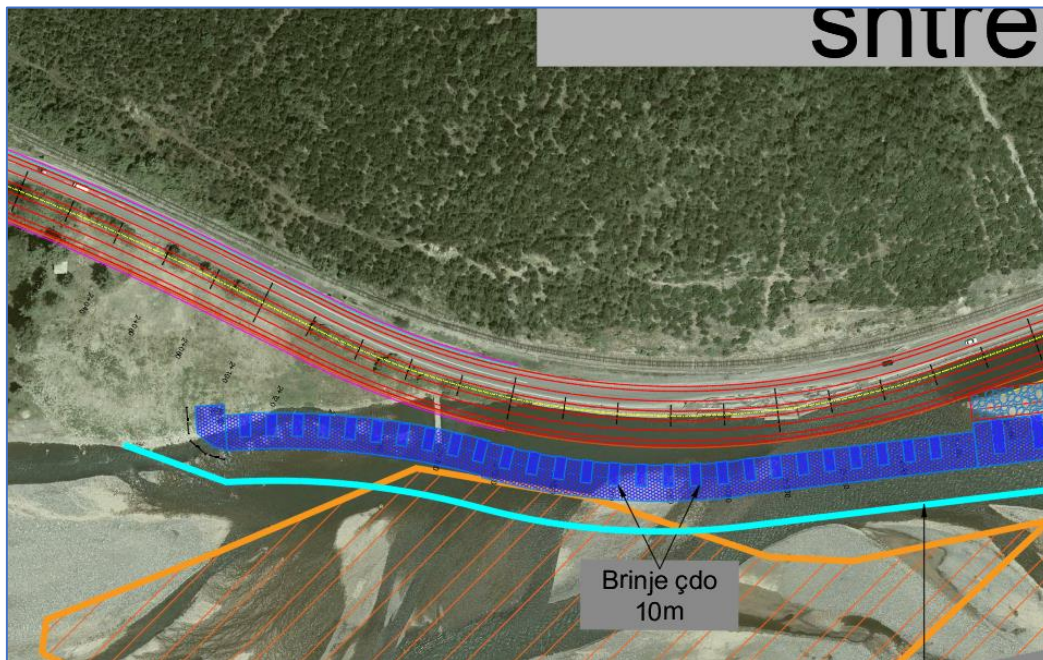
Planimetria e Mbrojtjes Lumore ne km 2+100 deri km 2+367
