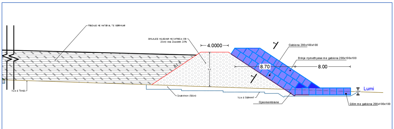
Profili Tip ne km 2+367 deri km 3+275
