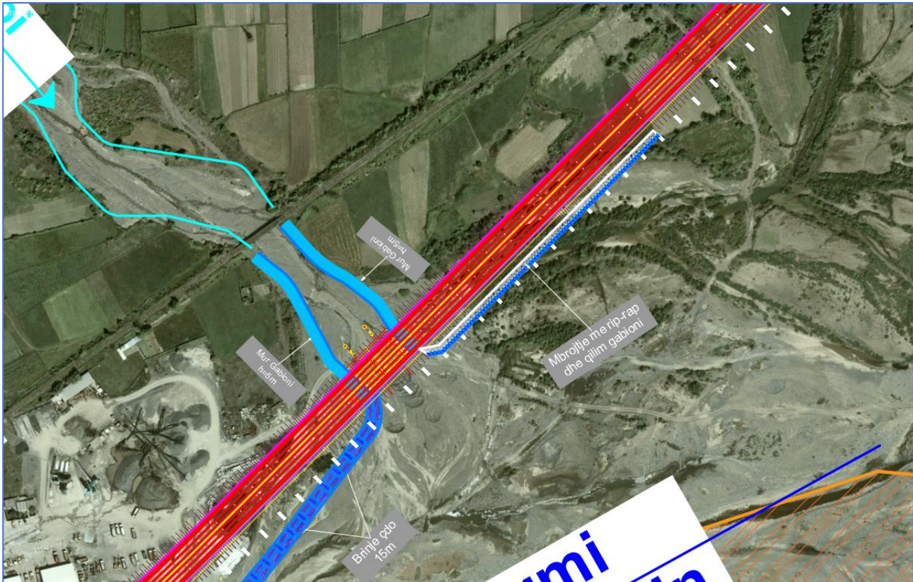
Planimetria e Mbrojtjes Lumore ne km 4+350 deri km 4+600
